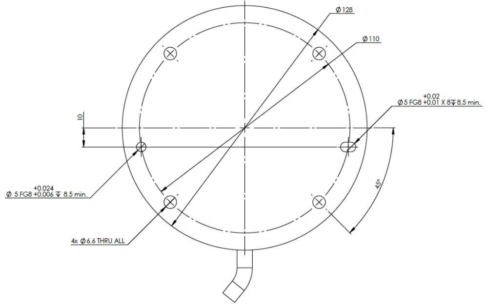
1.1: Robot tabanının alttan görünümü
